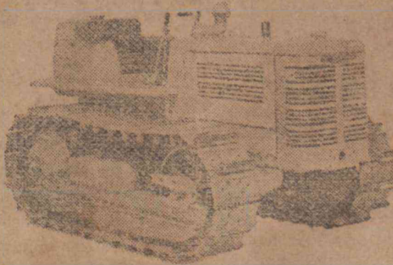
Tractor International Modelo T-6 para qualquer Alcool ou Kerosene, equipado com motor de quatro cilindros desenvolvendo 31.63 H. P. na barra de tracção e 26.68 H. P. na polia.
