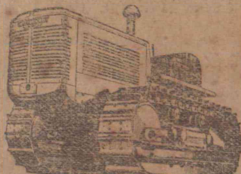
Modelo Internacional TD-18 com motor Diesel de 6 cilindros; desenvolve 72.38 H. P. (max.) na barra de tracção e 80.32 H. P. na polia.
