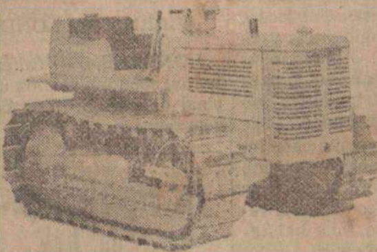
TracTractor International Modelo T-6 para queimar Alcool ou Kerosene, equipado com motor de quatro cylindros desenvolvendo 31.63 H. P. na barra de tracção e 36.68 H. P. na polia.
