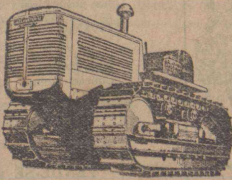
Modelo International TD-18 com motor Diesel de 6 cylindros; desenvolve 72.38 H. P. (max.) na barra de tracção e 80.32 H. P. na polia.
