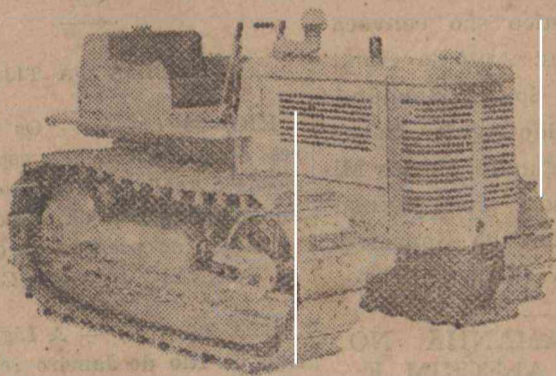
Tractor International Modelo T-6 para queimar Alcool ou Kerozene, equipado com motor de quatro cylindros desenvolvendo 31.63 H. P. na barra de tracção e 36.68 H. P. na polia.
