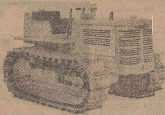
Tractor International Modelo T-6 para queimar Alcool ou Kerosene, equipado com motor de quatro cylindros desenvolvendo 31.63 H. P. na barra de tracção e 36.58 H. P. na polia.
