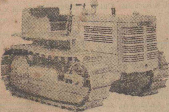
Tractor International Modelo T-6 para queimar Alcool ou Kerosene, equipado com motor de quatro cylindros desenvolvendo 31.63 H. P. na barra de tracção e 36.68 H. P. na polia.
